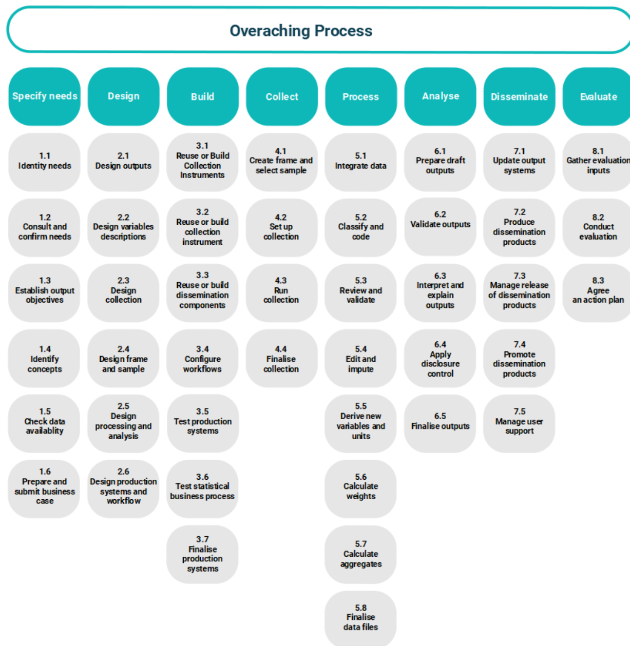
Fig. 6.1: GSBPM
