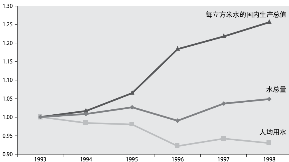
图九.1 1993年至1998年博茨瓦纳的用水、人口和国内生产总值指数
